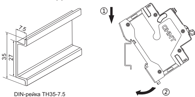
DIN-рейка TH35-7.5
