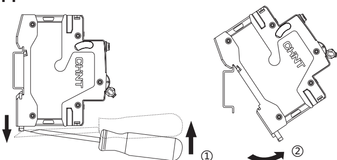
DIN-рейка TH35-7.5
